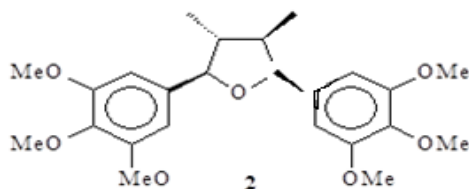
Epigrandisina (3)
